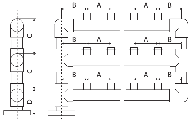
BATERIAS 3 FILAS
