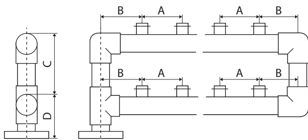
BATERIAS 2 FILAS
